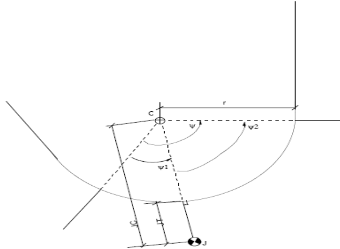
Figura 3 - llogaritja e SEL, hapi 1.
