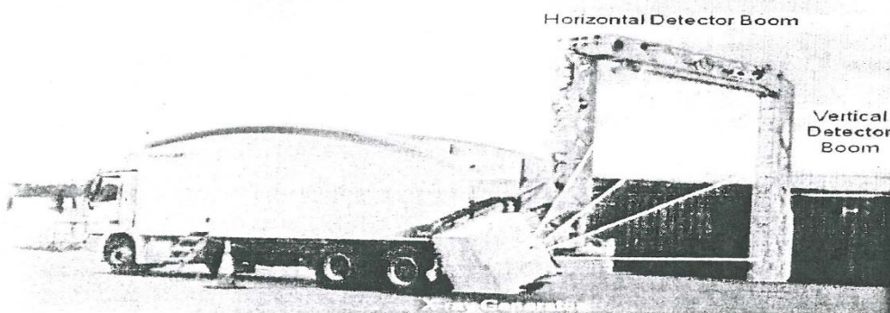
Figura 3. Eagle M60 – Sistemi imazhit me rreze X
