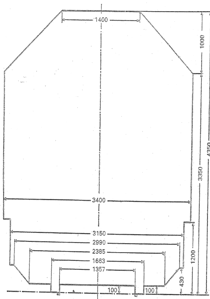
Gabariti i ngarkesës i pranuar nga C (NSB)
