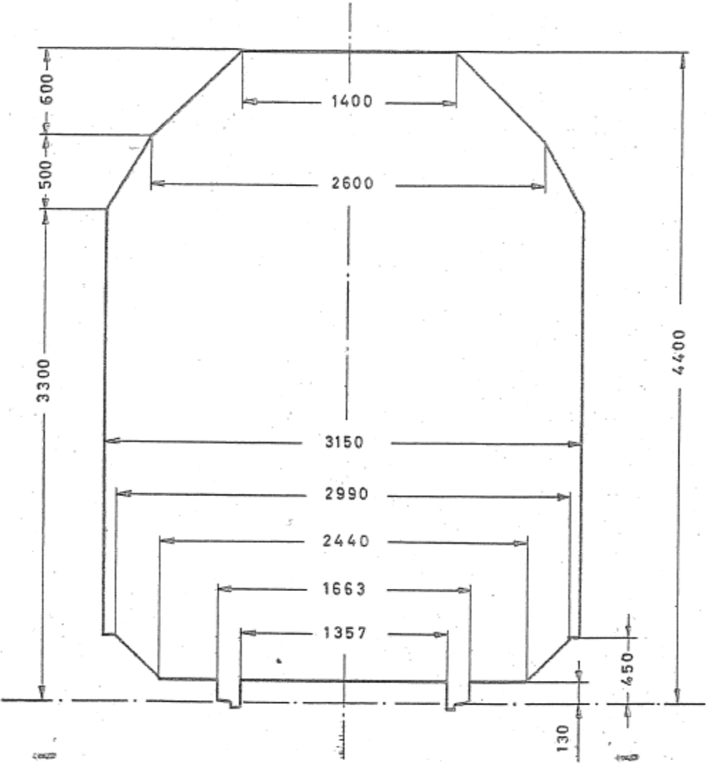
Gabariti i ngarkesës i pranuar nga RAI
