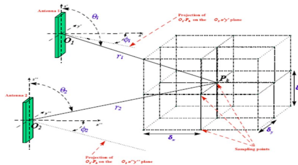
Figura 9: Fusha elektromagnetike rezultante e një sistemi antenash
