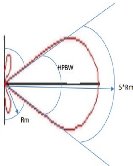
Figura 2.2: Paraqitje e Zonës së Kontrollit në planin horizontal
