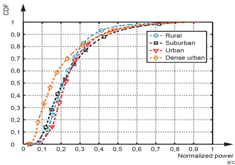
Figura 3.1: CDF-të empirike të fuqisë të transmetuar (të normalizuar) për mjedise të ndryshme në rrjetin 3G në Indi ([4] IEC TR 62669:2019, faqe 40)
