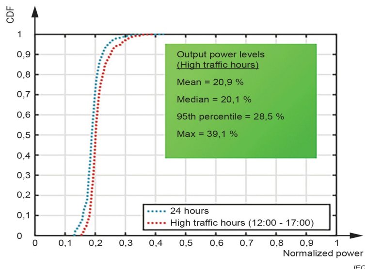
Figura 3.2: CDF-të empirike të fuqisë së transmetuar (të normalizuar) të kombinuar për një rrjet 2G/3G/4G në Suedi ([4], IEC TR 62669:2019, faqe 40)
