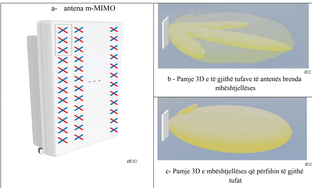
Figura 4: Antena e tipit massive MIMO dhe tufave elementare korresponduese së bashku me mbështjellësen e tyre
