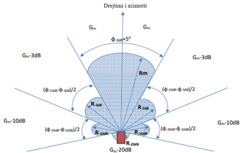
Figura 2.4: Skicë e zonave ku akses publik është i ndaluar në planin horizontal
