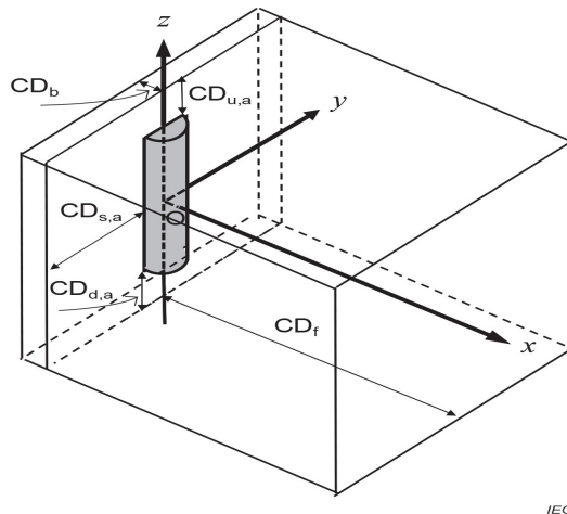
Figura 3: Kufiri i pajtueshmërisë – Zona Kritike në formë paralelepipedi
