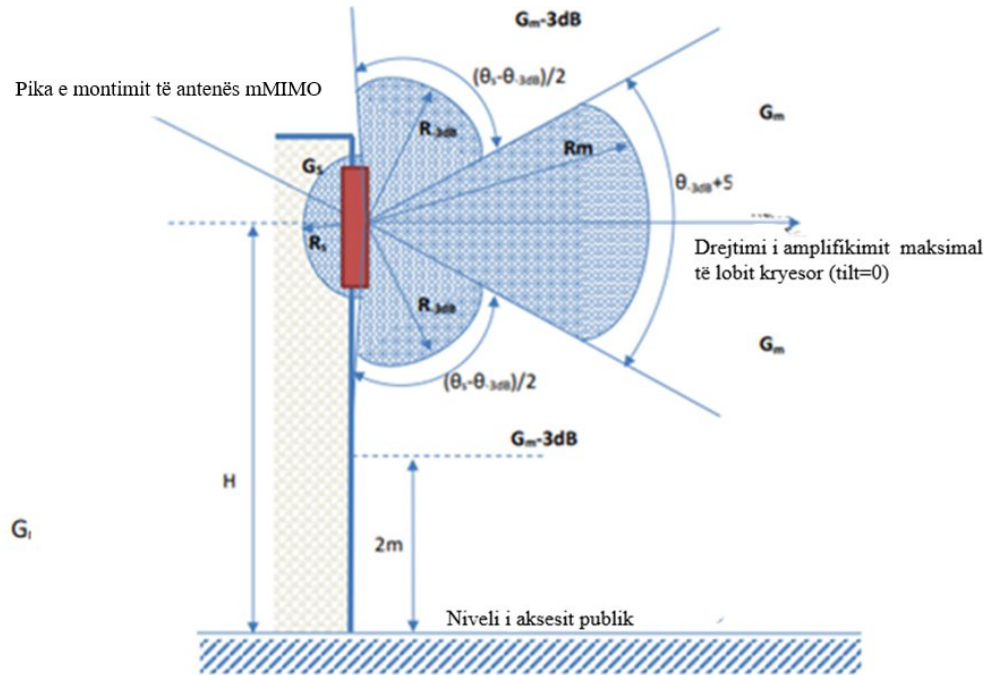
Figura 2.3: Skicë e zonave ku akses publik është i ndaluar në planin vertikal
