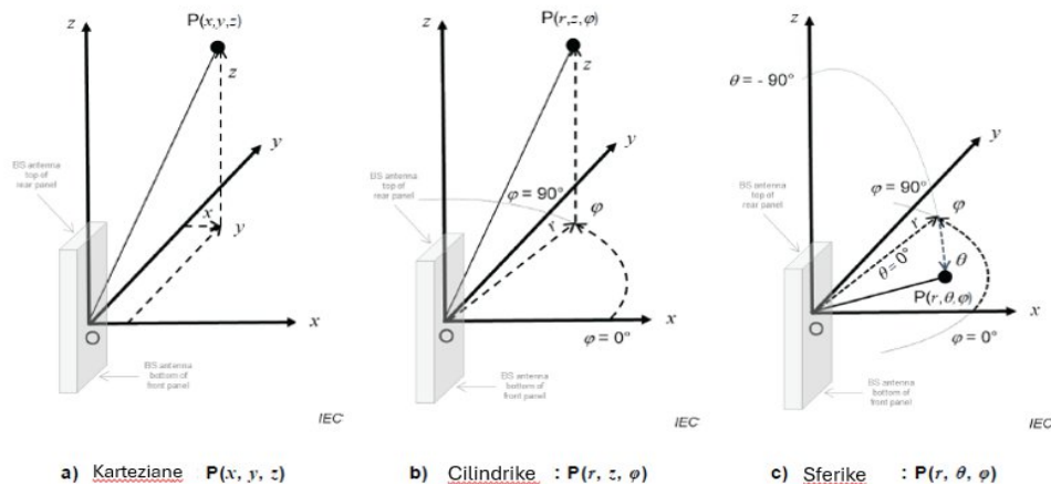
Figura 6: Sistemet e koordinatave karteziane, cilindrike dhe sferike për antenat e stacioneve bazë
