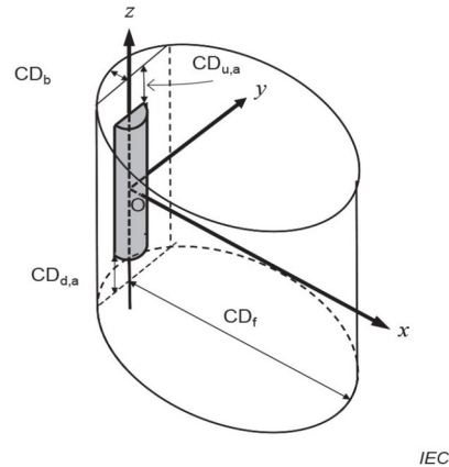
Figura 2: Kufiri i pajtueshmërisë – Zona Kritike në koordinata cilindrike
