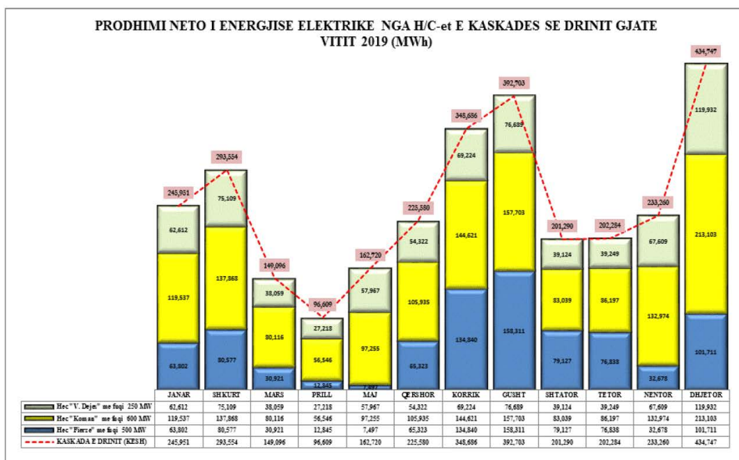
Figura 10 Prodhimi i Energjisë Elektrike nga HEC-et e Kaskadës së Drinit gjatë vitit 2019 (Burimi: KESH sh.a. , OST sh.a.).
