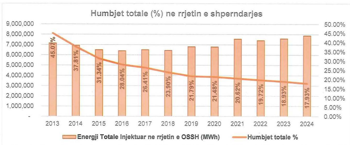
Figura 3. Humbjet (%) vjetore në rrjetin e shpërndarjes
