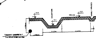
Prerja 1-1 Sh 1:200
