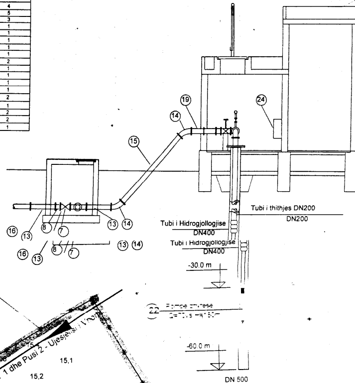
PRERJA B-B SKEMA TEKNOLOGJIKE SH 1:50
