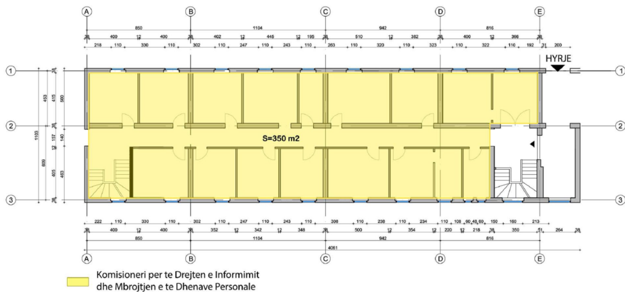
PLAN I KATIT PERDHE ( Kati i Pare )
