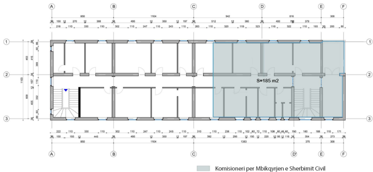
PLAN I KATIT TE PARE ( Kati i Dyte )
