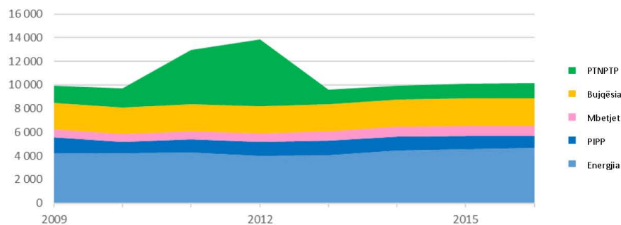
Figura 2. Niveli mesatar vjetor i emetimeve të GES në Shqipëri (kt CO 2 e), sipas sektorit (2009-2016)
