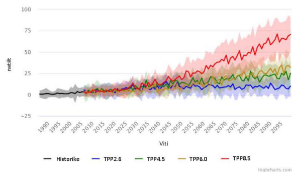
Figura 65. Netët tropikale (>20°C) në Shqipëri (1986-2099)
