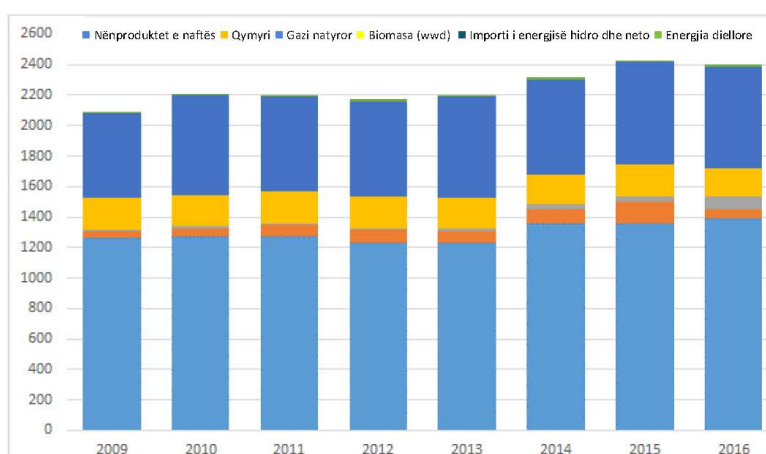
Figura 10. Furnizimi me energji (ktoe) sipas burimit të energjisë për periudhën 2009-2016
