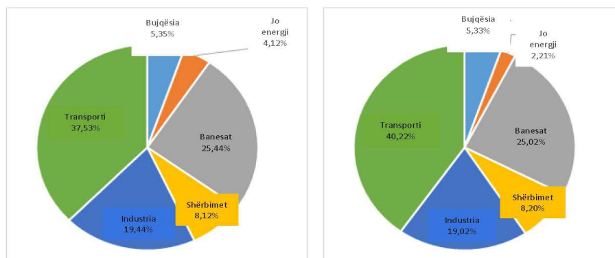
Figura 12. Konsumi final i energjisë sipas burimit të energjisë për vitin 2009 (%) dhe 2016 (%)
