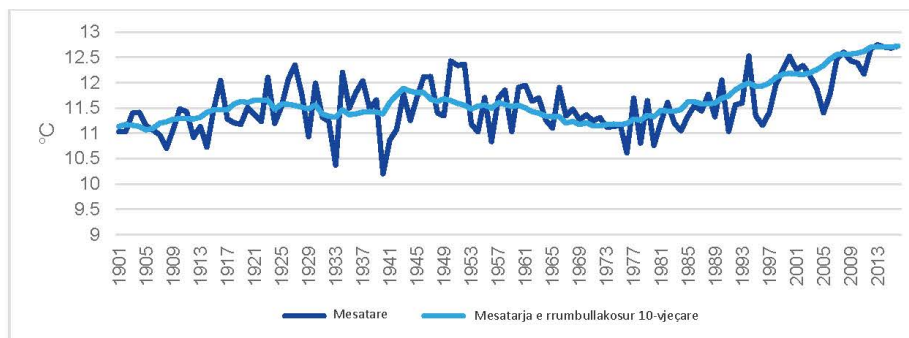
Figura 63. Temperatura mesatare vjetore dhe temperatura mesatare e rumbullakosur 10-vjeçare për Shqipërinë (1901-2016)
