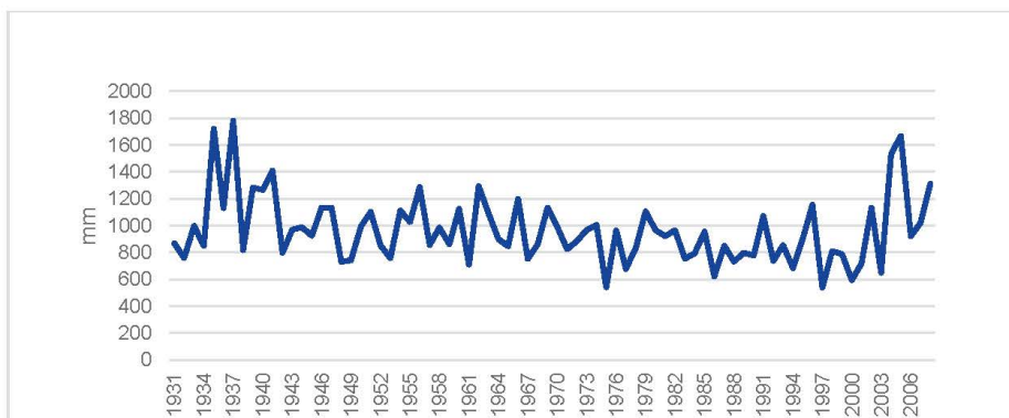
Figura 67. Reshjet mesatare për Vlorën (1931-2007)
