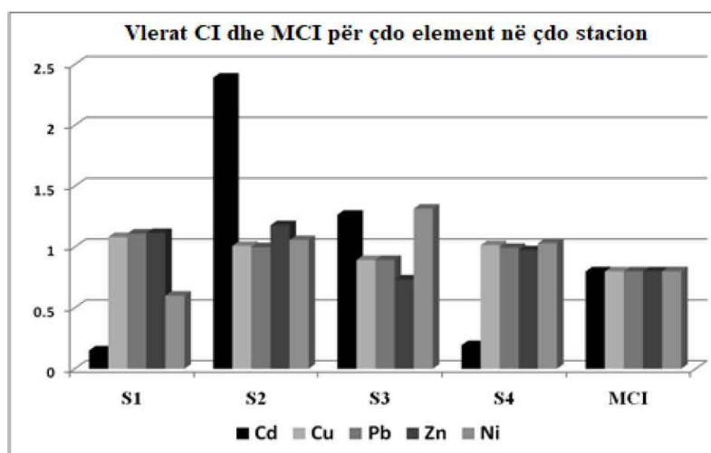
Figura 3 - Vlerat CI dhe MCI për çdo element
