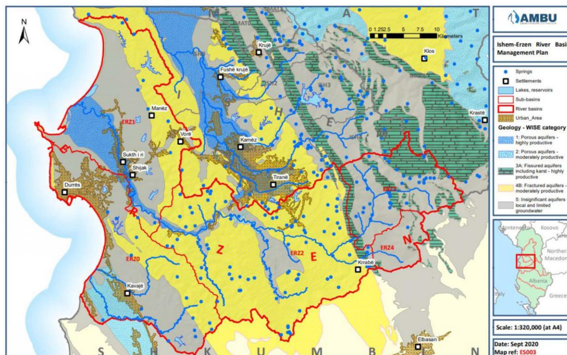
Harta 4-2 – Formacionet Kryesore Hidrojgeologjike
