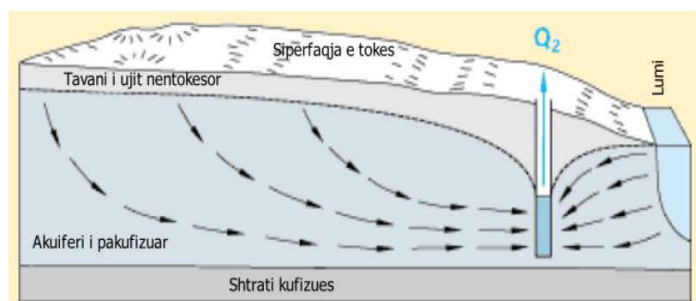
Figura 3-4 - Shembulli i Pakësimit të Prurjes Sipërfaqësore për Shkak të Nxjerrjes së Ujërave Nëntokësore
