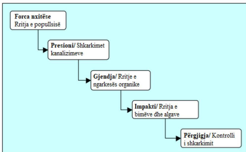
Figura 2 - Një ilustrim i kornizës analitike DPSIR
