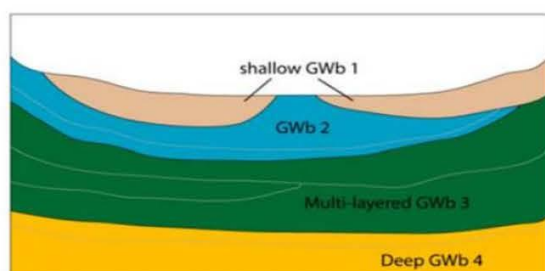
Figura 6-1- Ilustrimi i Trupave Ujqorë të Shumtë brenda një Akuiferi të Vetëm
