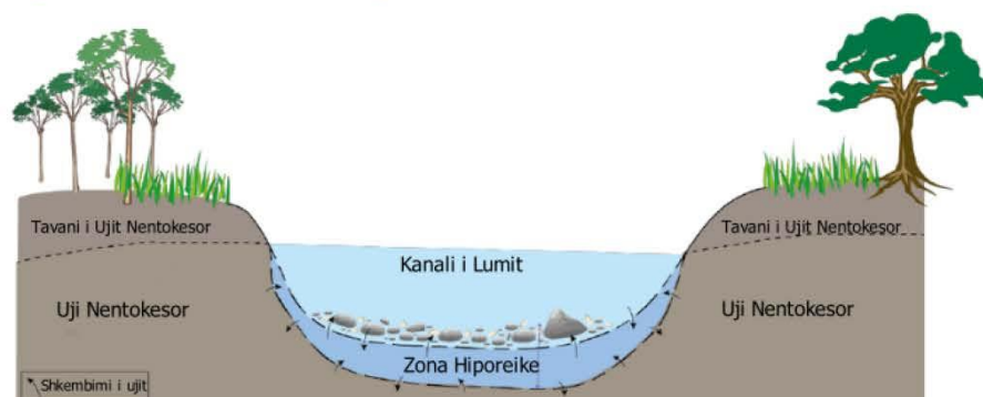
Figura 3-5 - Ilustrimi i Zonës Hiporike
