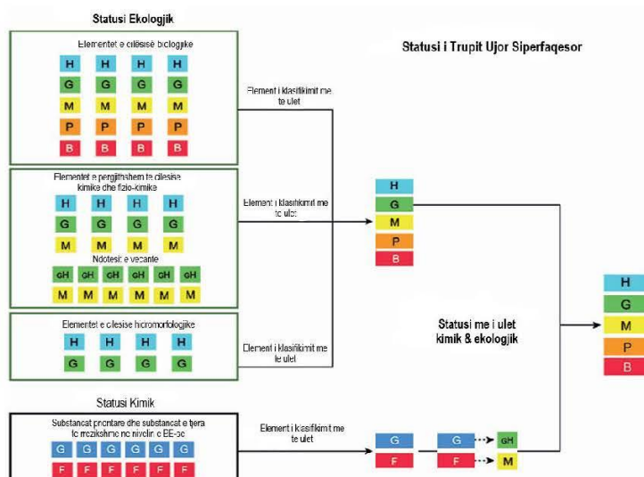
Figura 3-3- Procedura për Përcaktimin e Statusit të Përgjithshëm të Trupit Uhor
