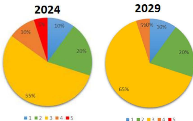
Figura 13-2 - Përqindjet Aktuale dhe të Parashikuara të Statusit të Trupave Ujorë Sipërfaqësorë
