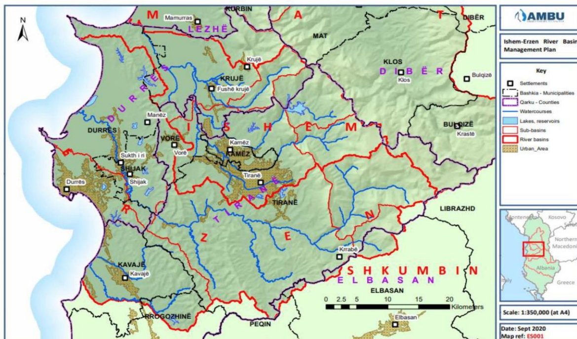
Harta 1-1 –Shtirja e Baseneve Ujore të Lumit Ishëm dhe Erzen
