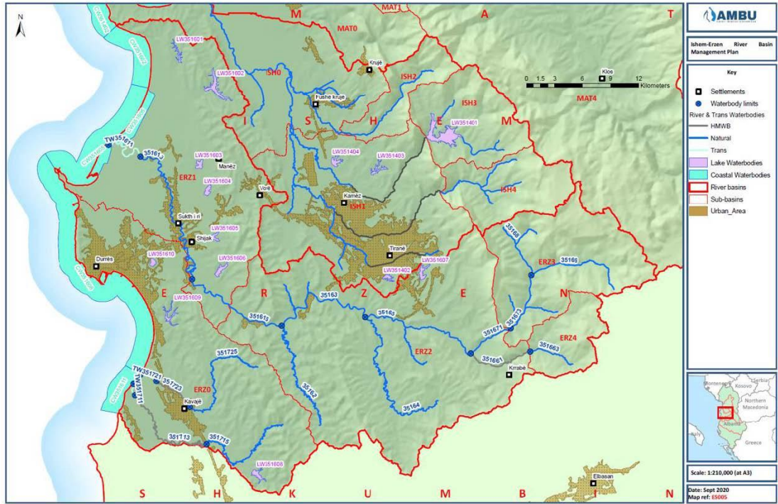
Figura 3-1- Kategoritë dhe përcaktimi i trupave ujorë sipërfaqësorë, baseni Erzen
