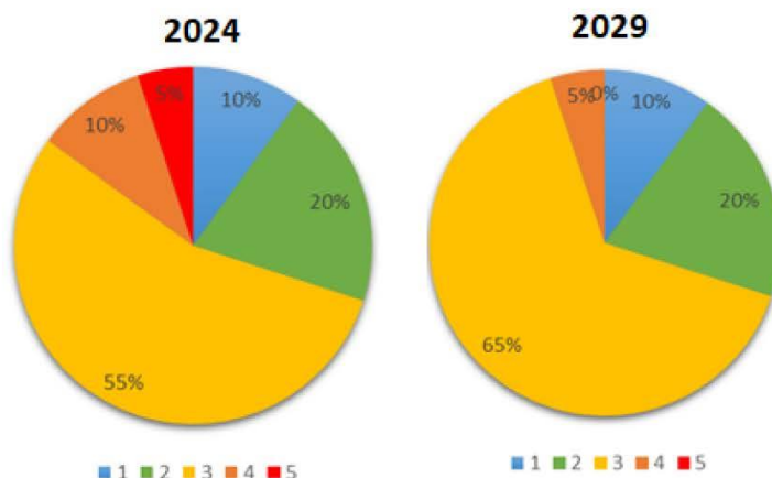
Figura2: Përqindjet aktuale dhe të parashikuara të statusit të trupave uJORë sipërfaqësorë
