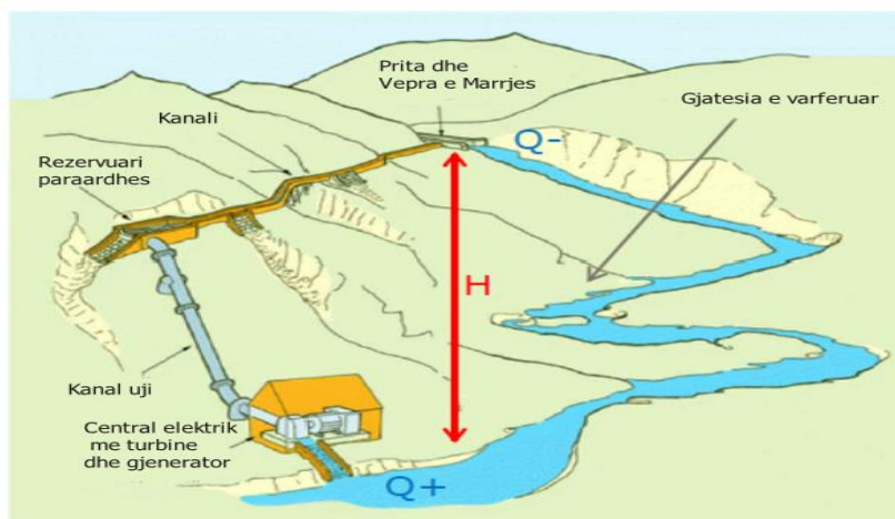
Figura 3-3 – Koncepti i Zonës së Shfrytëzimit nga Hidrocentralet
