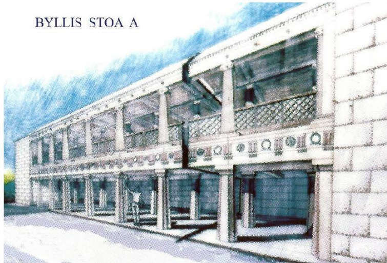
FIGURA 53 - STOA A E BYLLISIT. RIKONSTRUKSION VIRTUAL I KRAHUT LINDOR TË MONUMENTIT NGA N. CEKA-S.ÇELA
