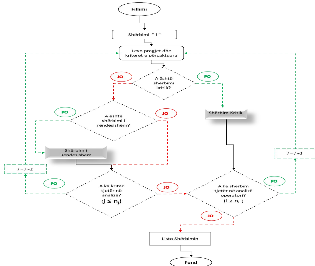
Figura 27. Skema logjike – OSE
