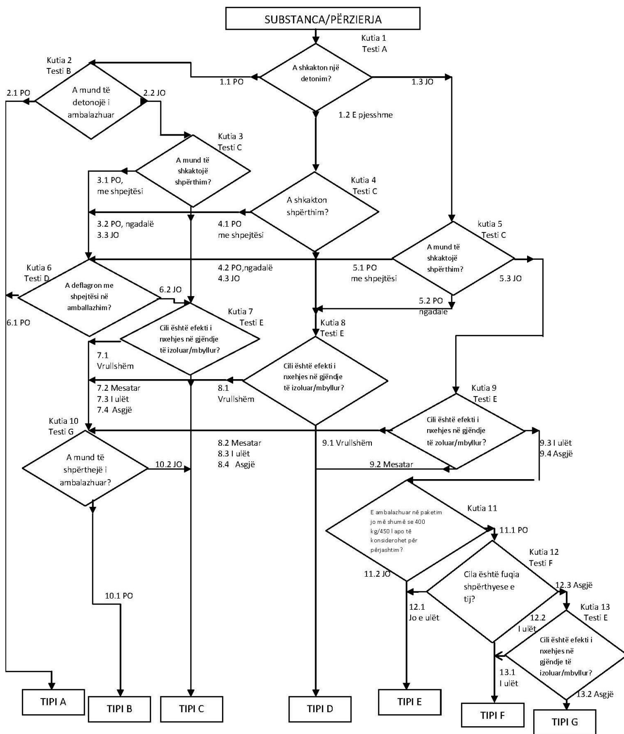
Figura 2.15.1 Peroksidet Organike
