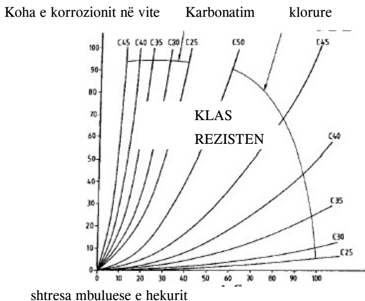
Figura nr. 8: Diagrama e jetës në punë të betonit
