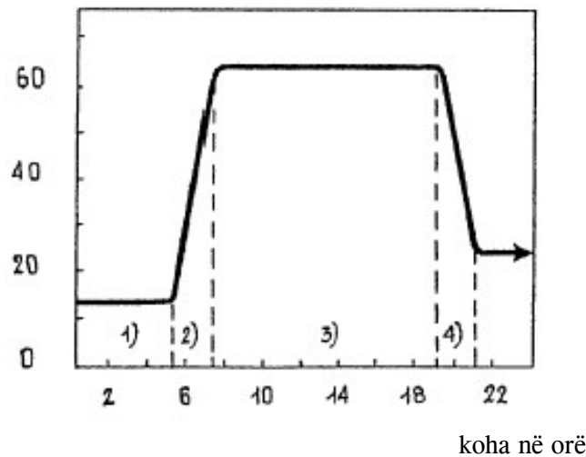
Figura nr.7 Shembulli i staxhionimit me avull me presion të zakonshëm (temperatura fillestare e brumit 13 °C)
