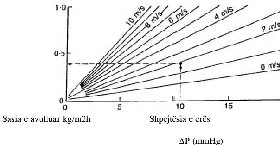
Figura nr.4: Shpejtësia e avullimit në funksion të shpejtësisë së erës dhe presionit parcial të avullit
