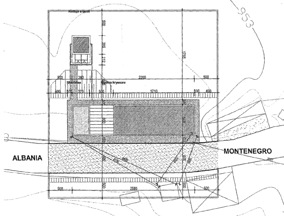
SKEMA E VENDOSJES TE SHESHIT NE RAJON SH 1:2000
