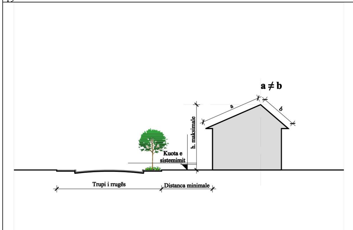
3.5 Lartësia maksimale e lejuar në metra e strukturës me mbulesë të pjerrët në terren të sheshtë, a \neq b
