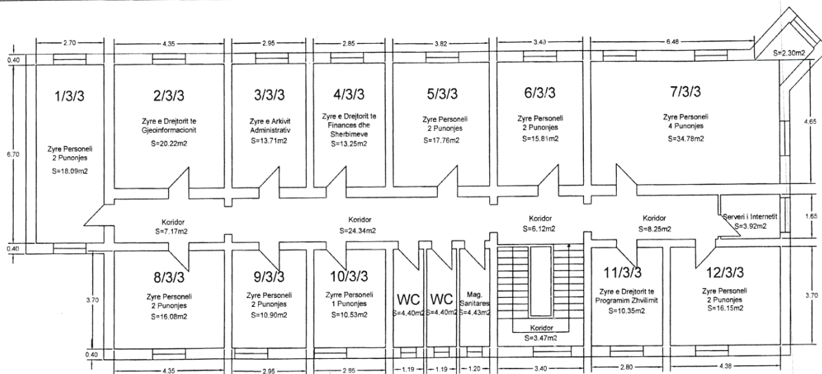
Planimetria e katit te III te Godines Qendrore te Sh.Gj.Sh rr. Kavajes
