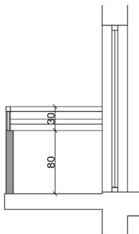
Figura 8. Prerje terthortë ballkoni
