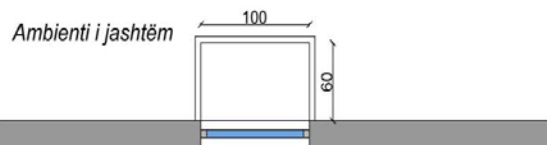
Figura 3. Ballkon me përmasa minimale
