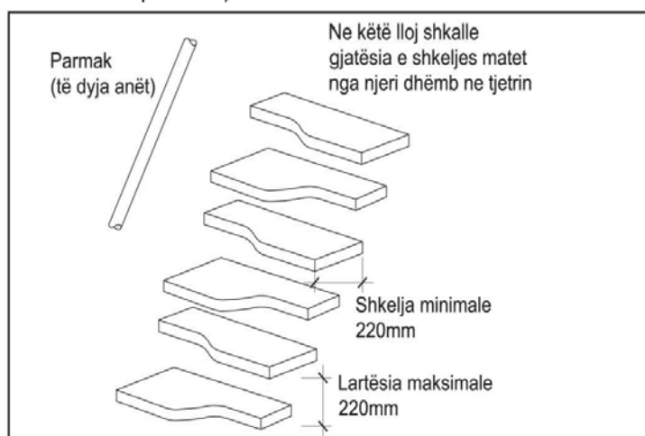
Figura 9 – Shkalië (me shkallare) me shkelje të ndryshueshme
