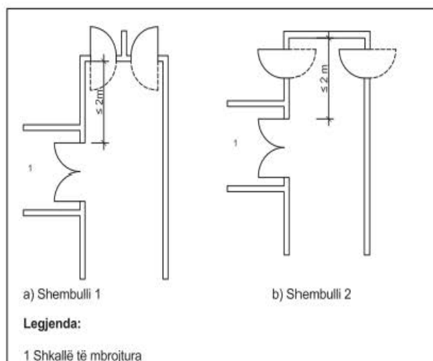
Figura 8 - zgjerimet e korridoreve përmes hapësirës së shkallëve të mbrojtura, gjerësia mund të reduktohet
