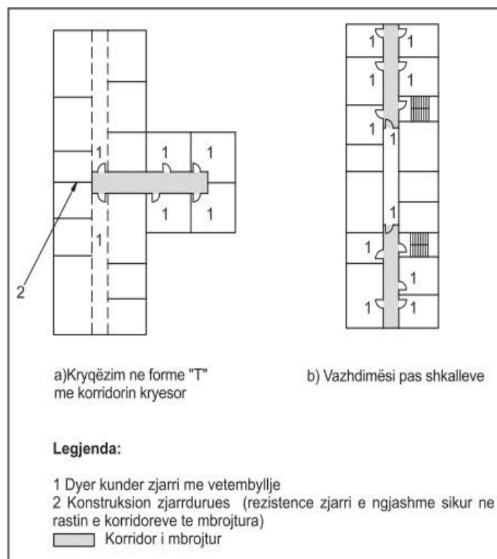
Figura 6. Koridoret pa dalje
