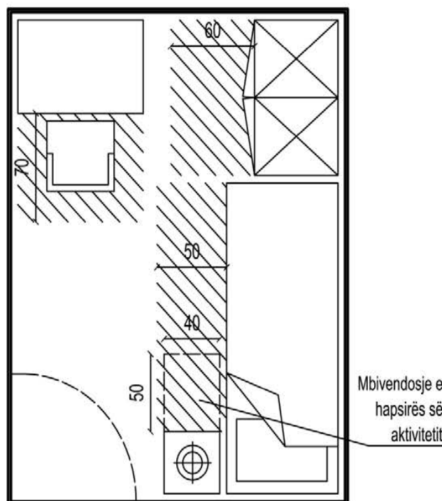
Fig. 7 Mbivendosje e hapësirës së aktivitetit në dhomë fjetieje për një person
