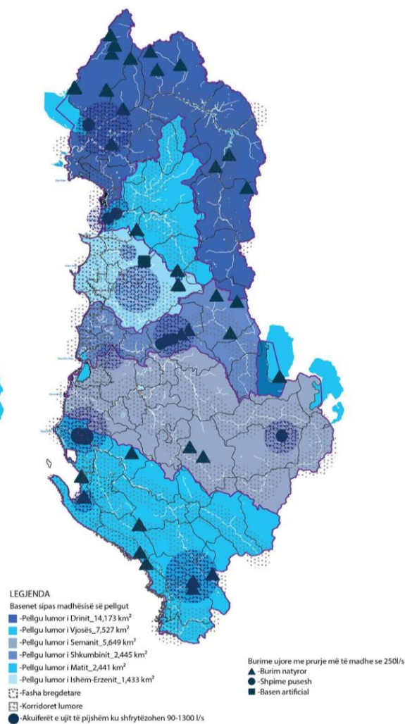
Harta 3.11 Basenet ujore sipas madhësisë së pellgut, ujëmbajtës dhe burimeve. Burimi: Raporti i gjendjes në mjedis, AKM; Pasuritë ujore të Shqipërisë, Niko Pano. Përpunoi: AKPT
