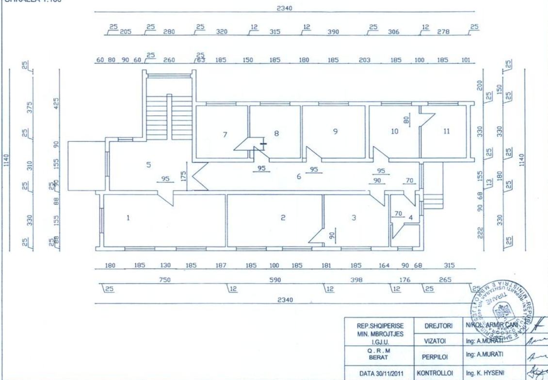
PLANIMETRIA E OBJEKTIT Nr.1 KATI I PARE SIP e Ndertimit = 198 m 2 SHKALLA 1:100
