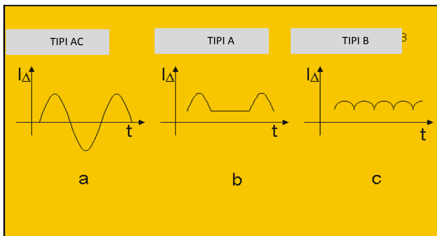
Figura 5. Tipat e dispozitivëve diferencialë në varësi të rrymës së veprimit ( I_{\Delta} )
