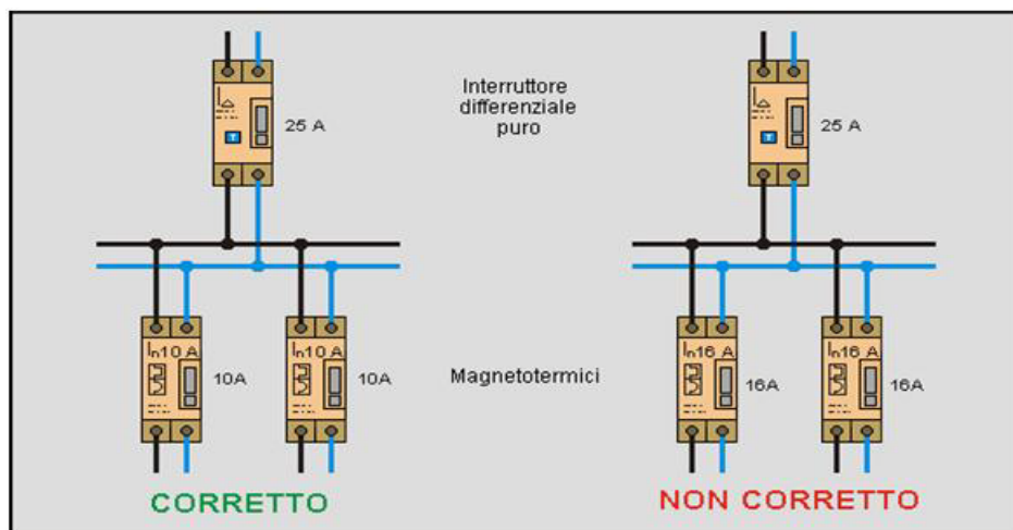
Figura 3. Shembull i koordinimit në mes të ndërprerësve dhe dispozitivit diferencial të pastër kundër mbingarkesës
