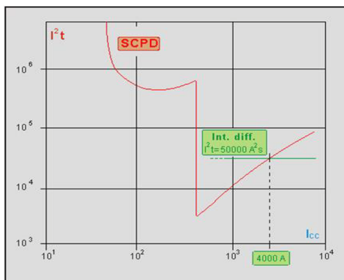
Figura 1. Koordinimi i dispozitivit diferencial me ndërprerësin. Verifikimi i I^2t
