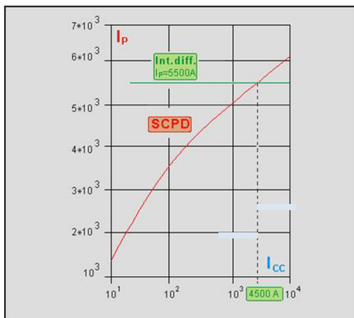
Figura 2. Koordinimi i dispozitivit të pastër kundër mbingarkesës
