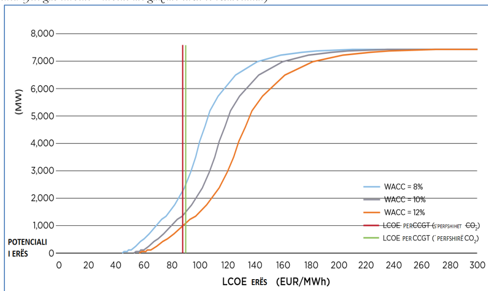
Figura 2: Potenciali i energjisë Eolike me kosto konkurruese në Shqipëri dhe LCOE
