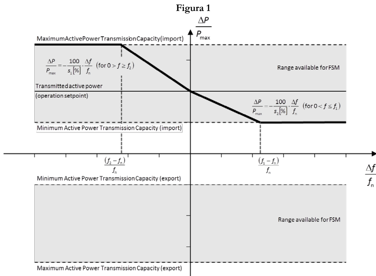
Figura 1: Aftësia e përgjigjes fuqisë aktive ndaj frekuencës së një sistemi HVDC në FSM duke ilustruar rastin me 0 deadbande dhe pandjeshmëri, me tarim pozitiv të fuqisë aktive (mënyra në import). \Delta P është ndryshimi e daljes së fuqisë aktive nga sistemit HVDC. f_n është targeti i frekuencës në rrjetin AC kur ofrohet shërbimi FSM dhe \Delta f është devijimi i frekuencës në rrjetin AC kur ofrohet shërbimi FSM.
