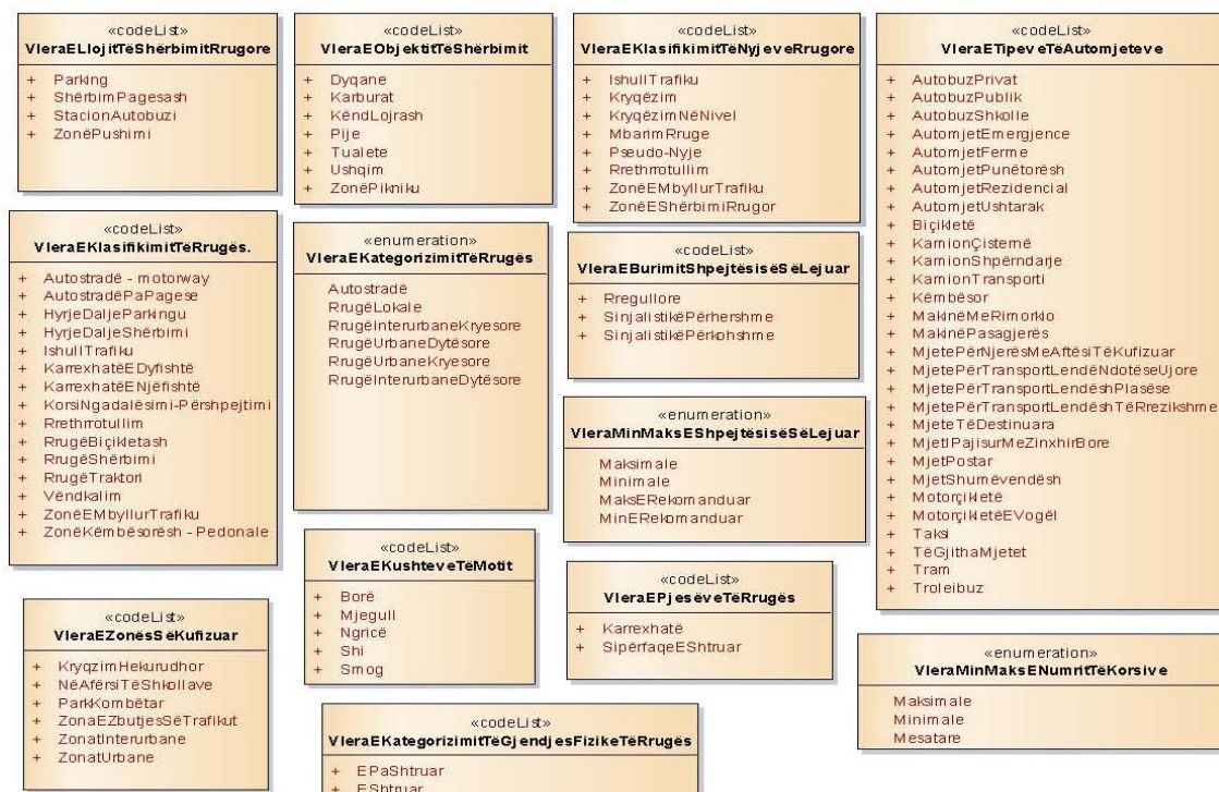
Figure 52: Rrjeti i Transportit Rrugor: Numërtimet dhe Kodlistat
