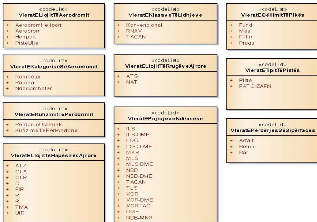
Figure 20: Rrjeti i Transportit Ajror : Numërtimet dhe Kod listat
