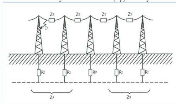
Figurë 17. Paraqitja e rezistencës që përfshihen në një lidhje me tokën
