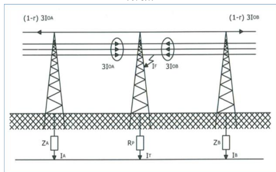
Figurë 16. Tokëzimi referues
