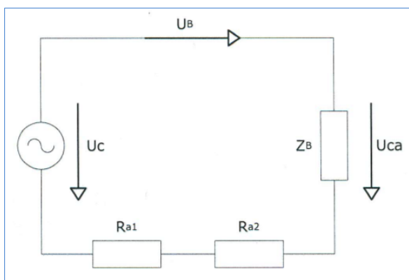
Figurë 14. Skema e qarkut të kontaktit
