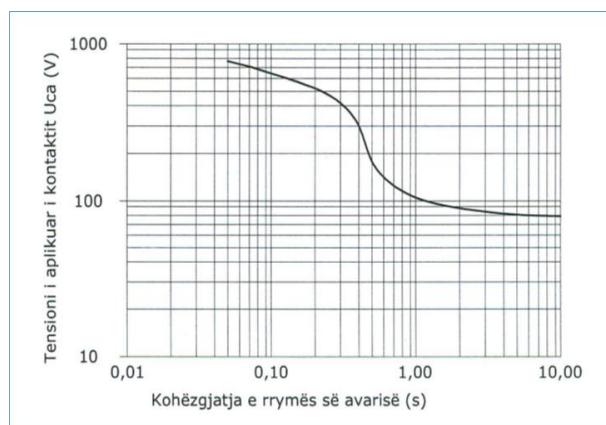
Figurë 13. Vlerat e tensionit të lejuar të kontaktit të aplikuar U_{ca} në varësi të kohëzgjatjes së rrymës
