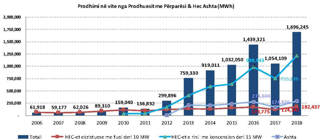
Figure 63 Ecuria e prodhimit nga prodhuesit me Përparësi & Hec Ashta (MWh) (Burimi OSHEE sh.a)
