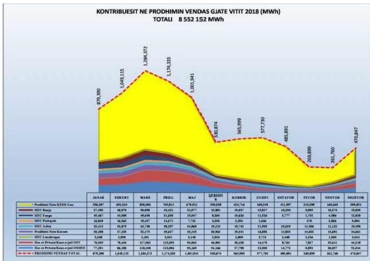
Figure 8 Kontribuesit në prodhimin vendas gjatë vitit 2018 (MWh)
