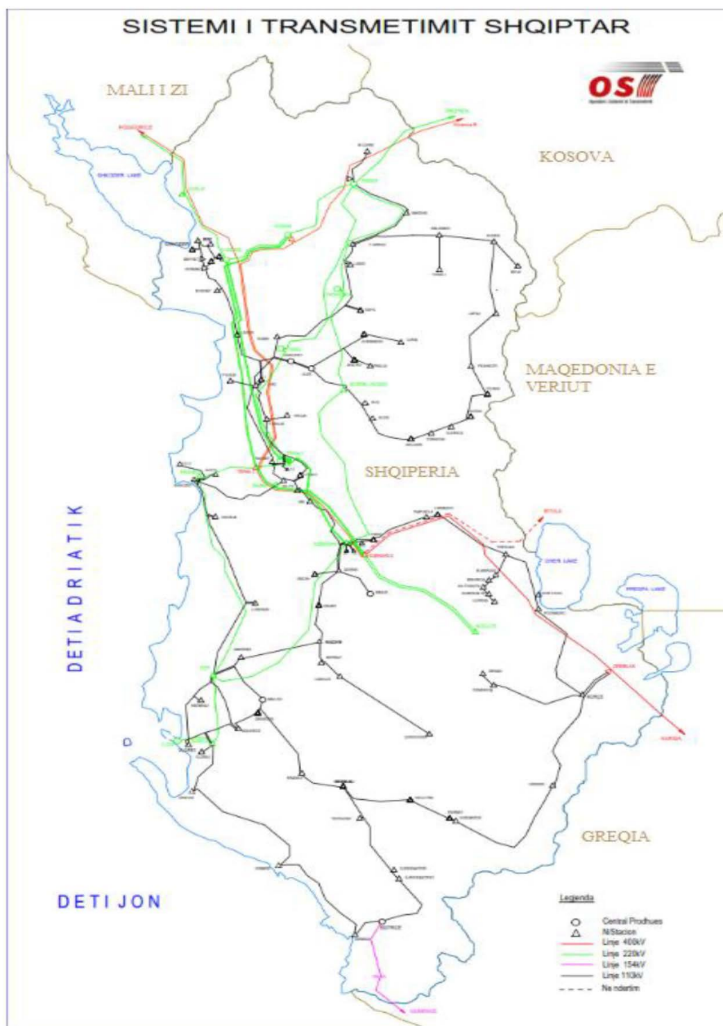
Figura 30 Harta e Sistemit të Transmetimit Shqiptar.
