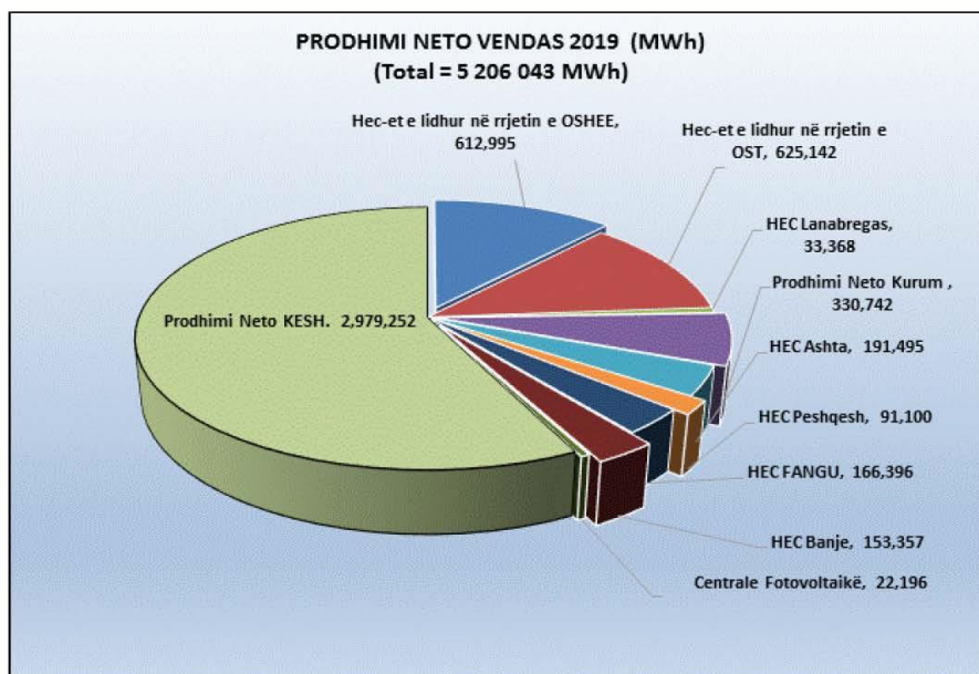
Figura 4 Prodhimi neto vendas për vitin 2019.
