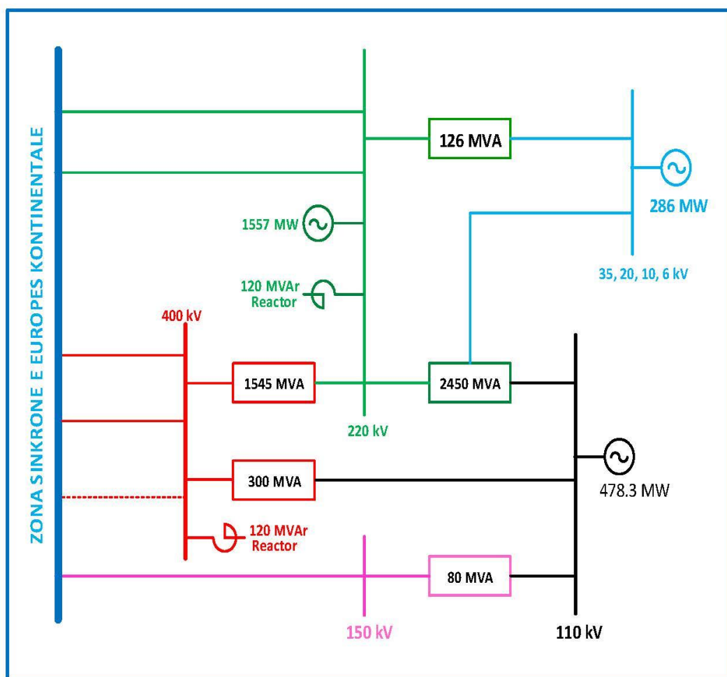
Figura 29 Struktura e Sistemit të Transmetimit të Shqipërisë.
