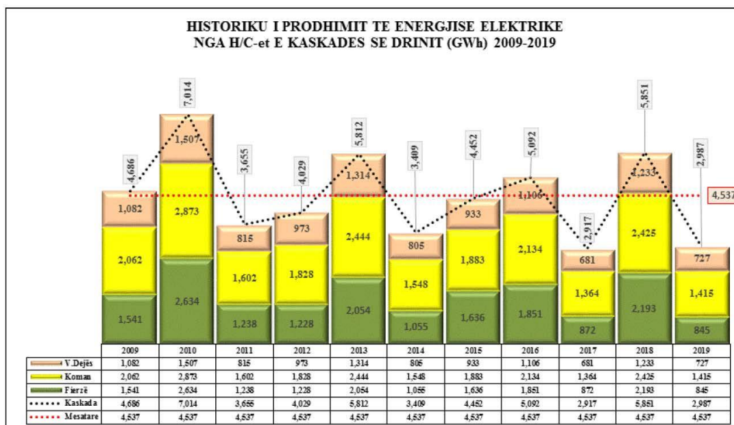
Figura 9 Historiku i Prodimit të Energjisë Elektrike nga HEC-et e Kaskadës së Drinit (Burimi: OST sh.a.).
