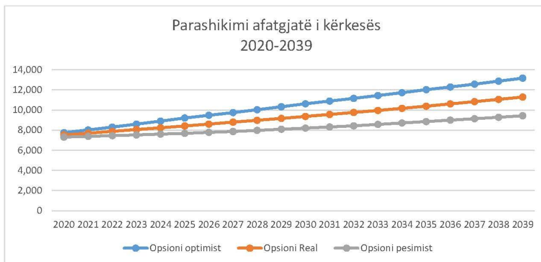
Figura 37 Parashikimi afatgjatë i kërkesës për energji elektrike për periudhën 2020 – 2039.
