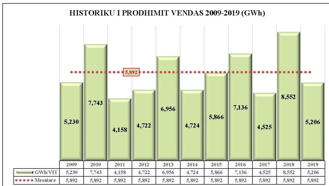
Figura 7 Prodhimi neto vendas historik për periudhën 2009-2019
