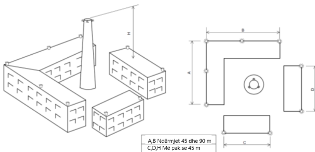
Figura A2-3. Ndriçim tipik i një grupi pengesash
