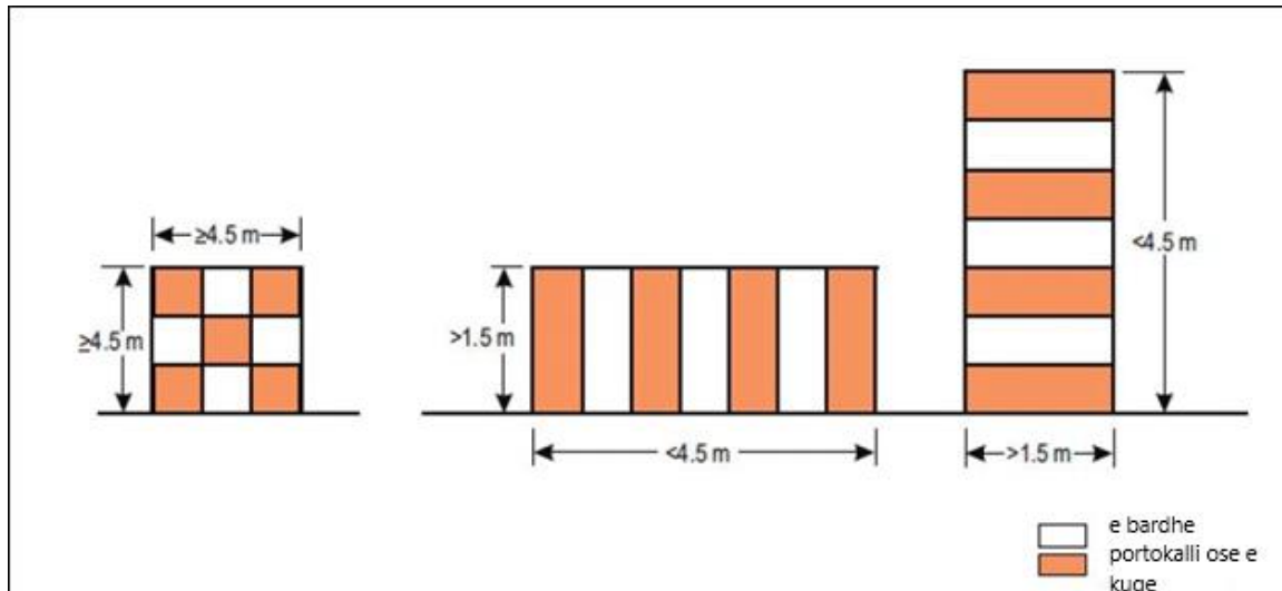
Figura A2-2. Shembuj të shënjimit dhe ndriçimit të strukturave të larta
