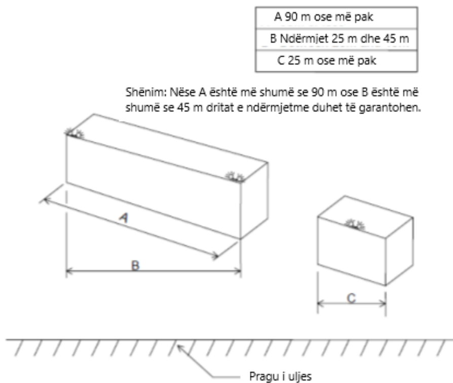
Figura A2-4. Ndriçimi tipik i pengesave të zgjeruara horizontalisht
