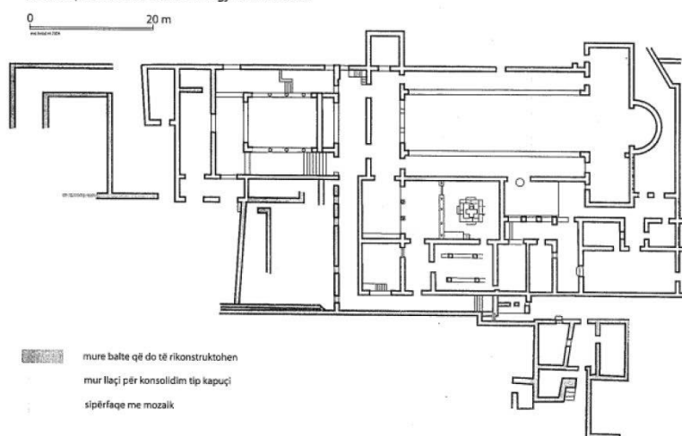
BYLIS - Planimetria e bazilikës B muret që do të konsolidohen gjatë vitit 2004
