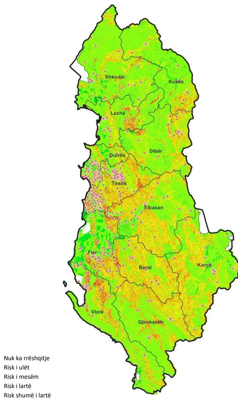
Fig. 26. Harta e ndjeshmërisë ndaj rrëshqitjeve e Shqipërisë (nga Shërbimi Gjeologjik Shqiptar)
