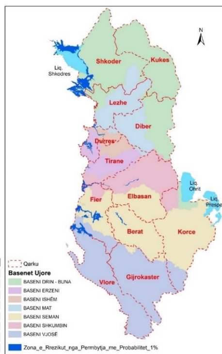
Fig. 21. Harta e rrezikut nga përmblytjet me periudhë kthimi 1 herë në 100-vjet
