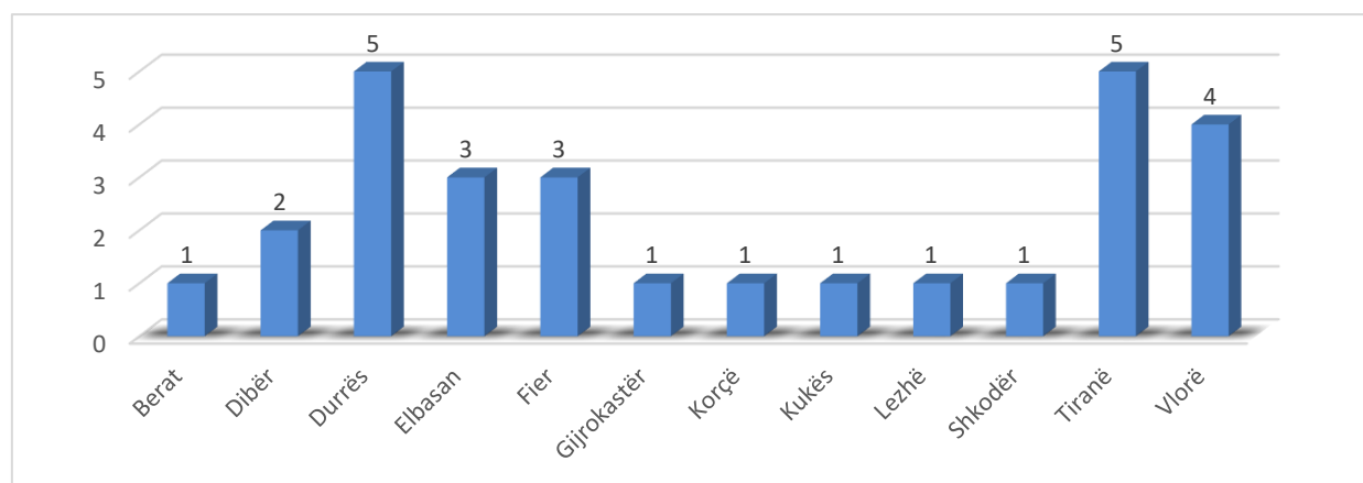
Fig. 19. Risku i tërmetejeve në qarqet e Shqipërisë
