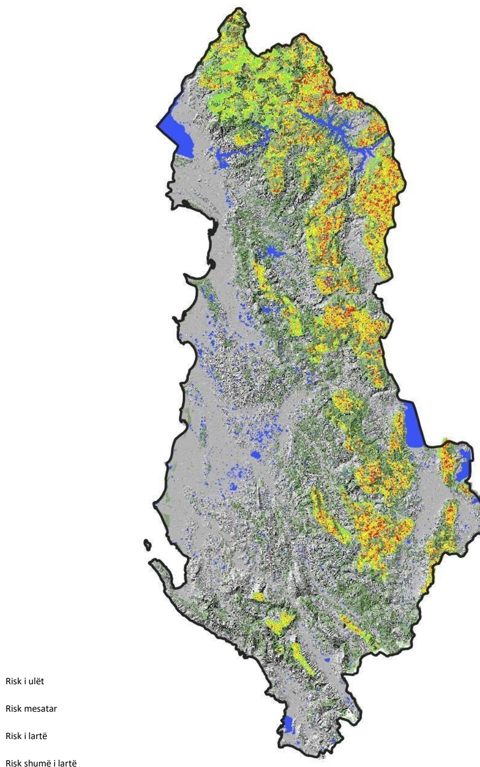
Fig. 27. Harta e ndjeshmërisë së ortekëve të Shqipërisë
