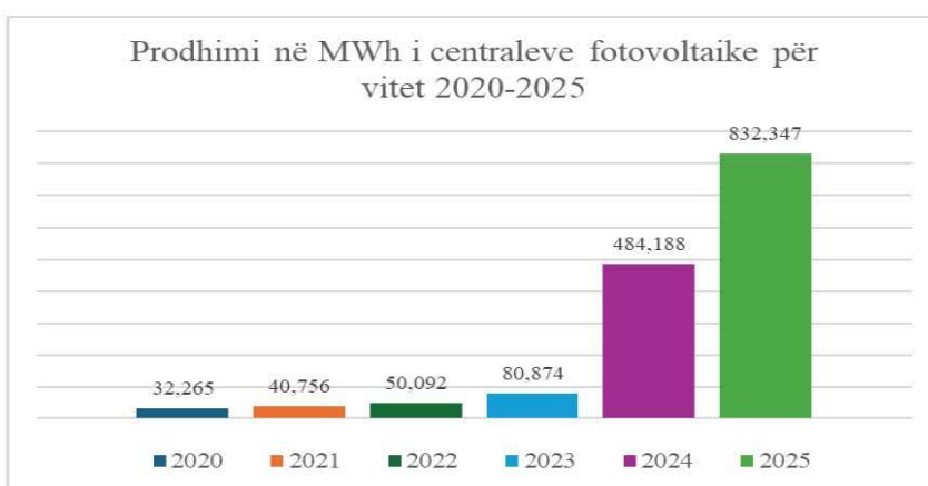
Figura 15. Prodhimi (MWh) i centraleve fotovoltaike për vitet 2020-2025
