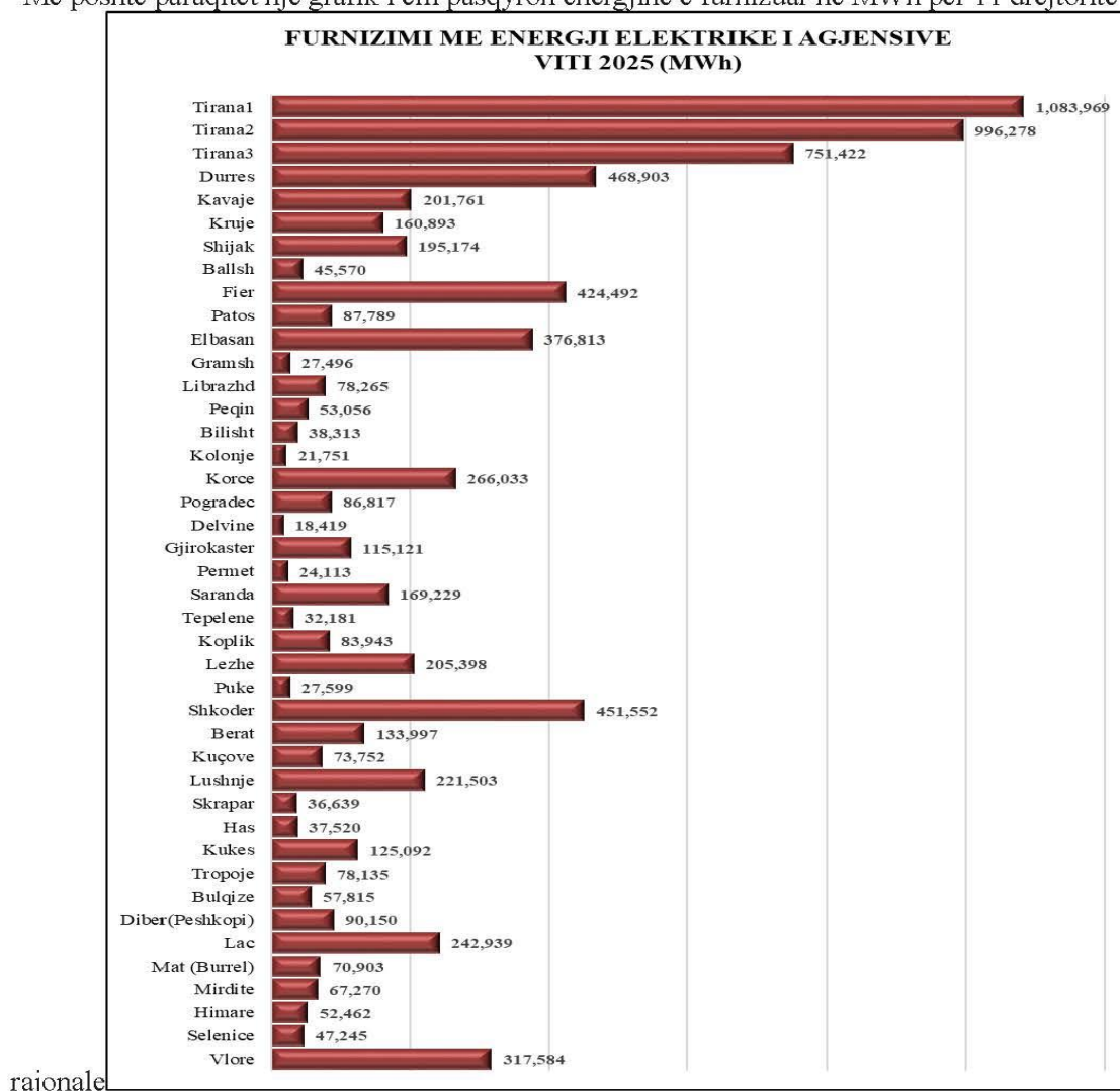
Figura 38. Furnizimi me energji elektrike të ndara sipas drejtorive rajonale në MWh për vitin 2025
