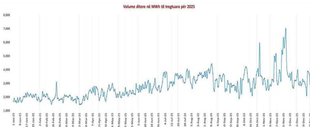
Figura 55. Volumet ditore mesatare të tregtuara për vitin 2025
