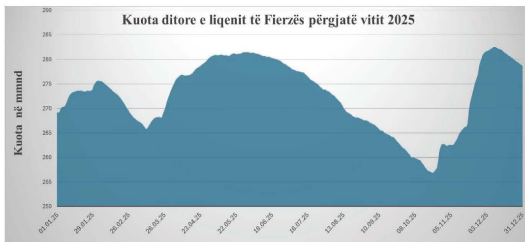
Figura 8. Niveli i Liqenit të Fierzës gjatë vitit 2025 (mmnd)
