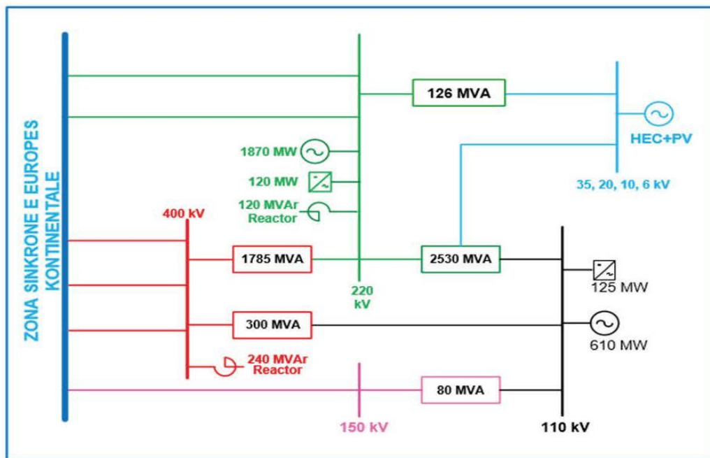
Figura 18. Struktura e Sistemit të Transmetimit të Shqipërisë
