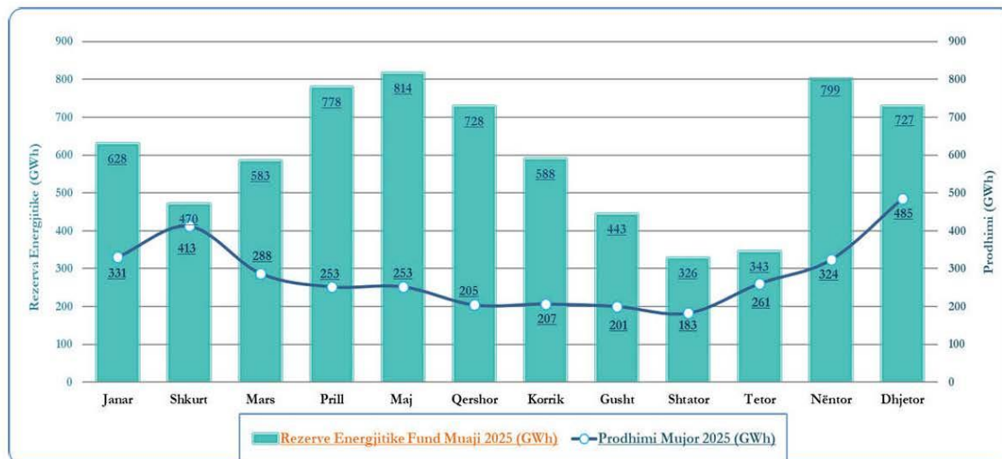
Figura 11. Rezerva energjetike çdo fund muaji dhe prodhimi mujor 2025 (GWh)
