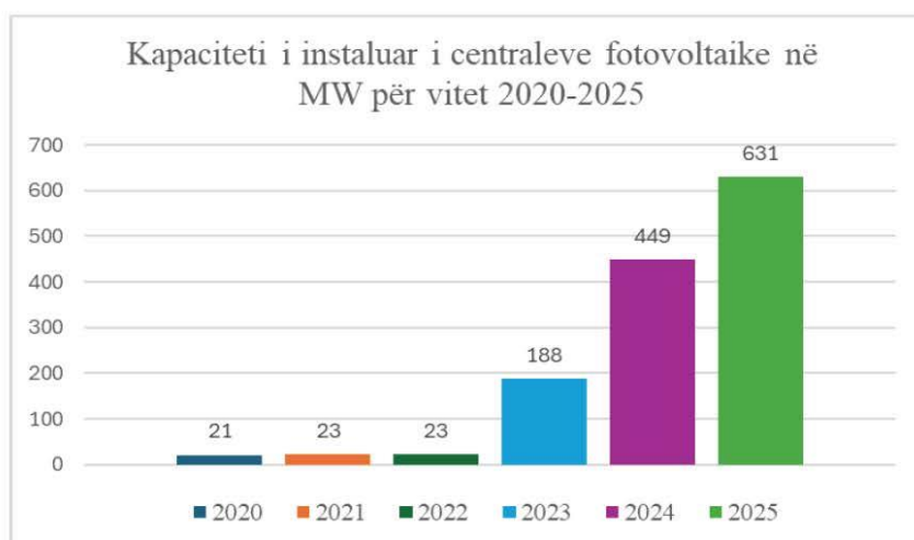
Figura 14. Kapaciteti i instaluar (MW) i centraleve fotovoltaike për vitet 2020-2025
