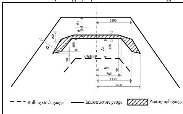
Figura C.3. Matës statik i pantografit për sistemin e matësit të gjurmës 1 520 mm
