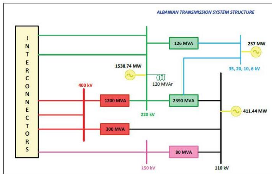
Figura 17: Skema e rrjetit të transmetimit në Shqipëri
